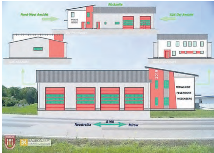
Bauzeichnung mit Ansicht von allen Seiten.
